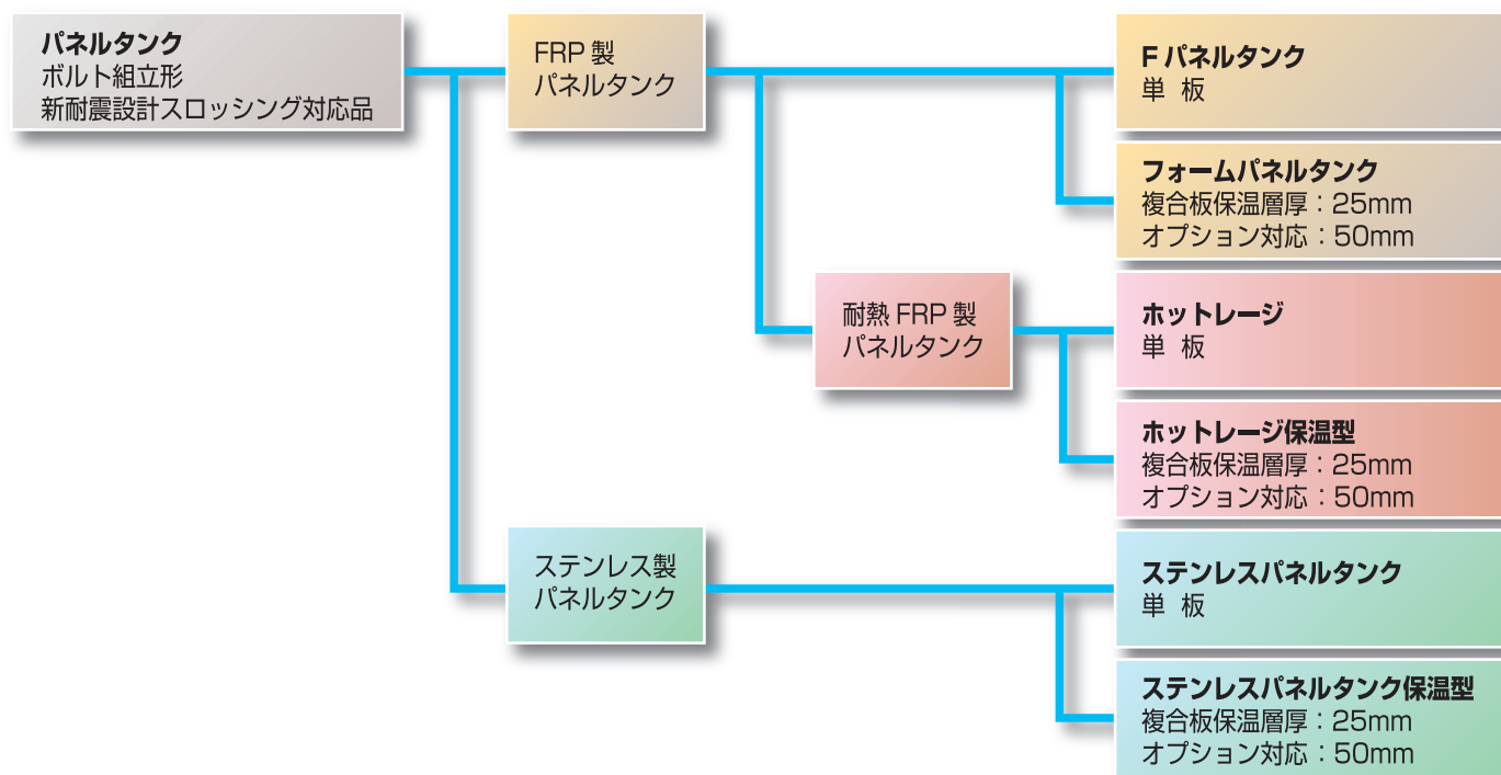
●FRP製パネルタンク
