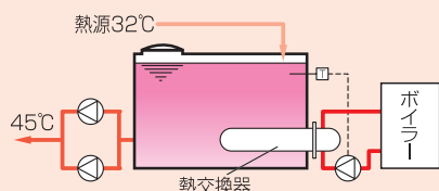
高温の熱源を有効利用するシステム例
