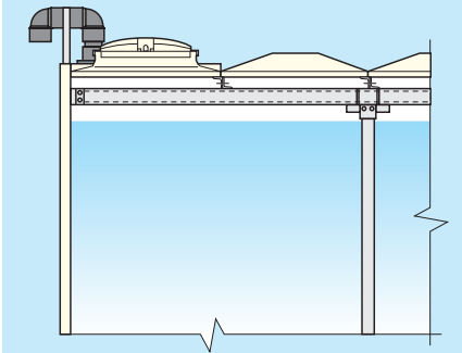
耐雪型構造例
