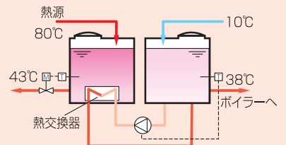
高温の熱源を有効利用するシステム例
