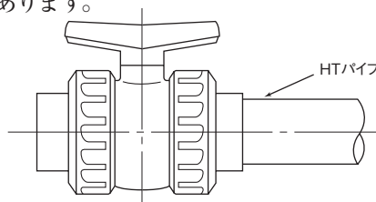
図-41 TS式バルブとの接続（φ13～φ100）
