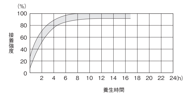
図-5 常温における接着強度と養生時間
