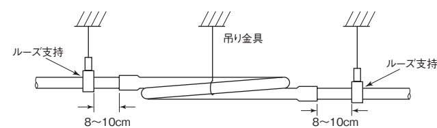
図-35 エキスパンション(伸縮継手)の水平取付け
