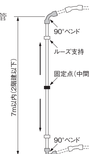
図-17 縦引配管の実例
