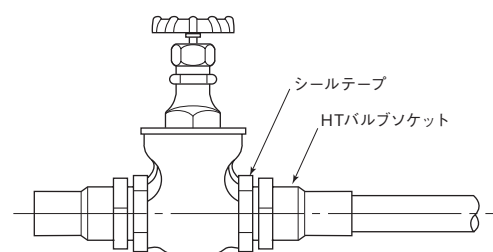
図-39 ねじ式バルブとの接続（φ13～φ50）
