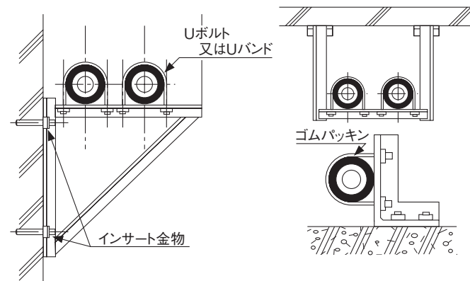
図-31 固定支持の方法
