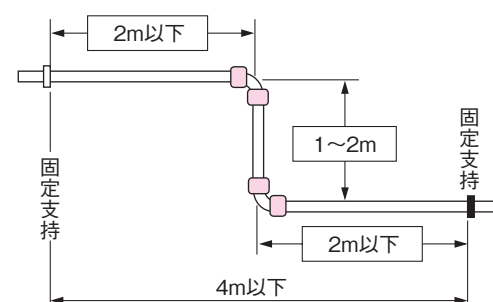
図-25 吊り配管実例（2）
