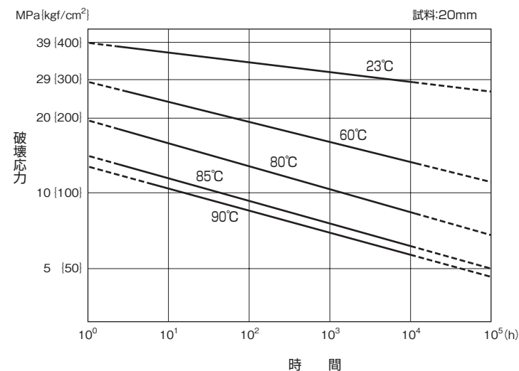
図-3 温度別長期内圧クリープ試験結果
