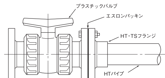
図-42 フランジ式バルブとの接続（φ13～φ100）
