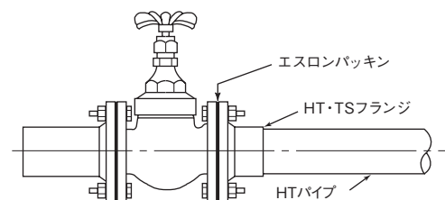
図-40 フランジ式バルブとの接続（φ13～φ100）
