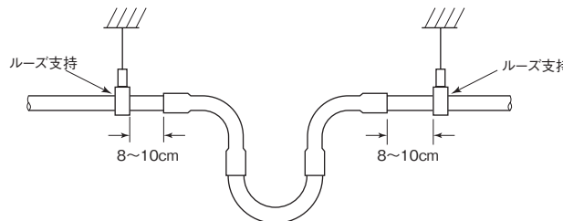
図-34 エキスパンション(伸縮継手)の下向き取付け
