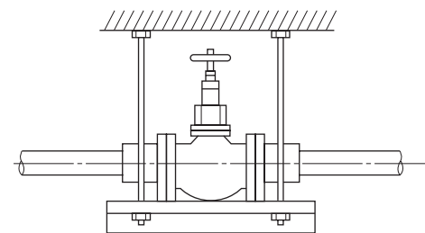
図-33 バルブの支持方法
