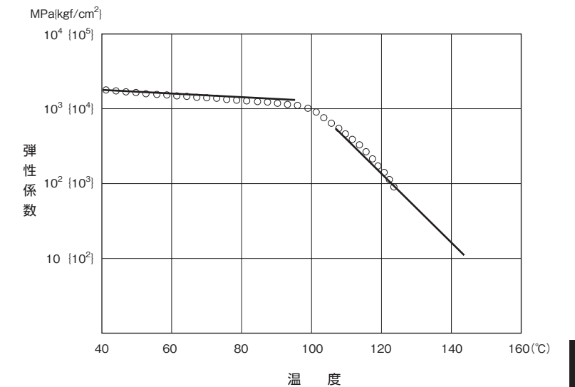
図-4 温度と縦弾性係数の関係
