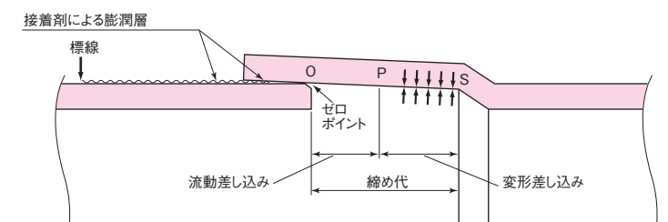
図-37 TS接続の原理
