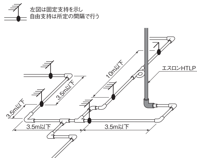
図-23 吊り配管略図
