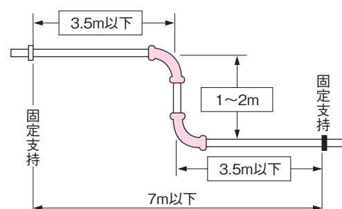
図-24 吊り配管実例（1）
