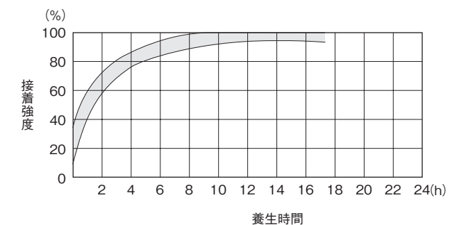
図-6 90℃における接着強度と養生時間
