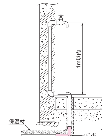
図-28 地中埋設配管実例(2)
