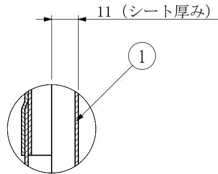
A部詳細
