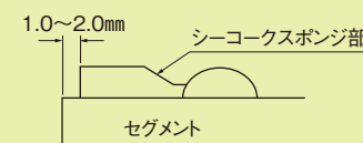
シーコークスポンジ部の先端部とセグメント内側の寸法
