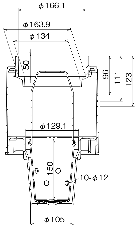
断面図A-A
