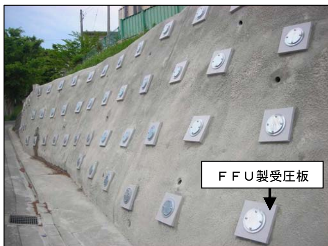
セキスイ合成木材(FFU)製受圧板 (KFFU低荷重用受圧板 K300S)
