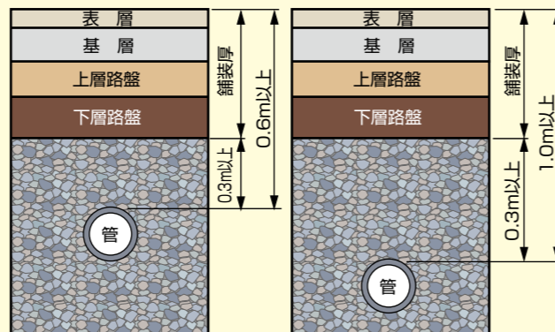
■ 本線以外の歩道の地下に設ける場合 ■ 本線の場合
