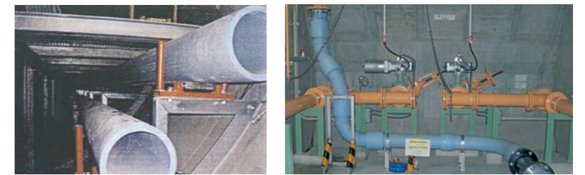
シールド内に設置された汚泥圧送管 処理場施設内に設置された汚泥配管
