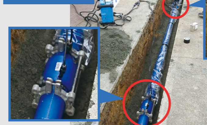
EFソケット+EFソケット 同時通電施工事例
