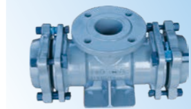
PメカチーズFS型 呼び径75~200×75
