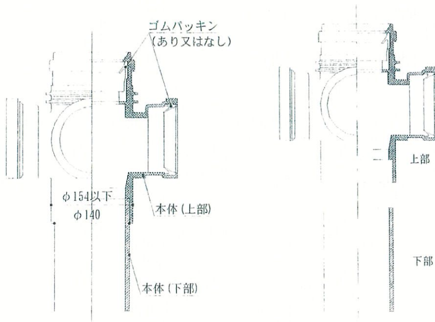
図4 樹脂製継手の構造例
