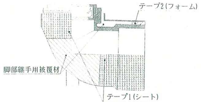
図9 脚部継手の構造例 (被覆材あり)
