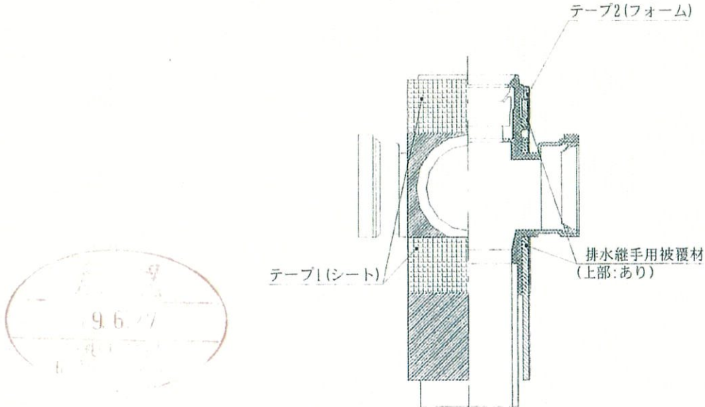
図3 排水継手の構造例
