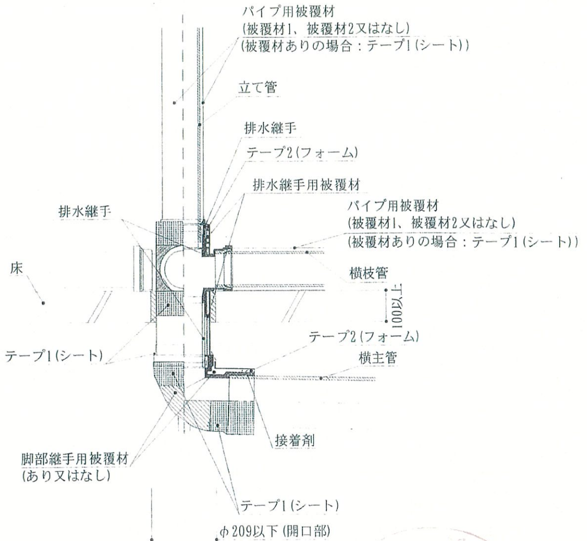
図1 配管の構造例
