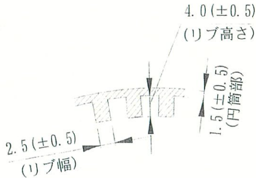
図 6 パイプ用被覆材 1 の断面構造例
