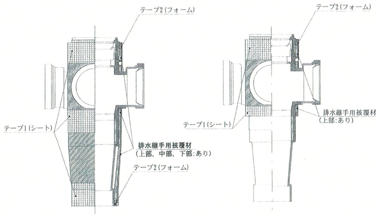
図5 排水継手の構造例（全体 被覆材）
