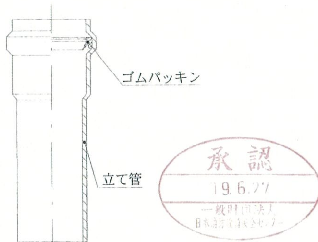
図9 立て管 (ゴムパッキン付き) の構造例
