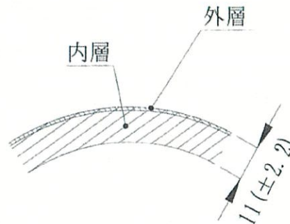
図 1 1 パイプ用被覆材 2 の断面構造例
