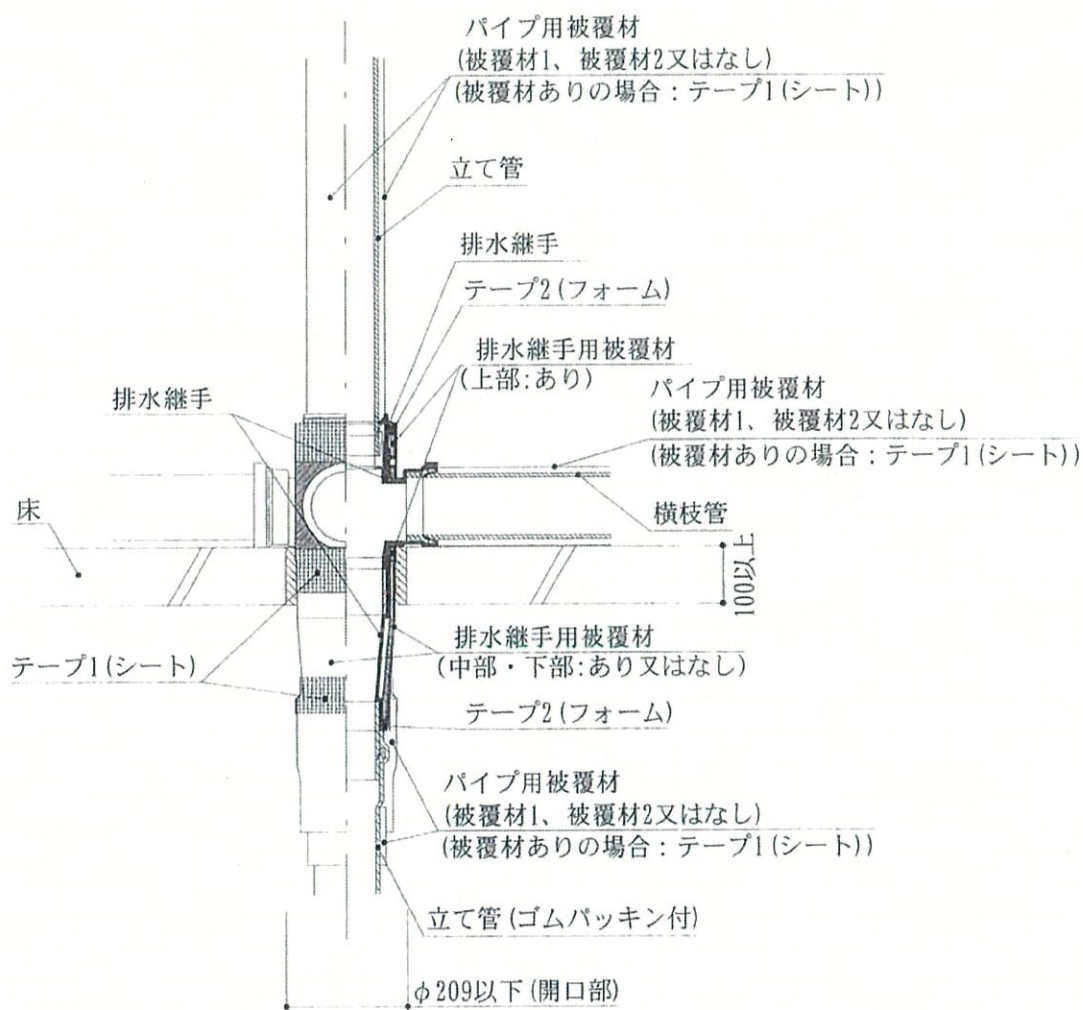
図14 施工図例 (脚部継手を接続しない場合)
