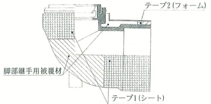
図13 脚部継手の構造例（被覆材あり）
