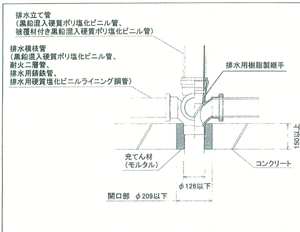
図1 断面図
