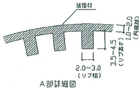
図4 被覆材の断面構造
