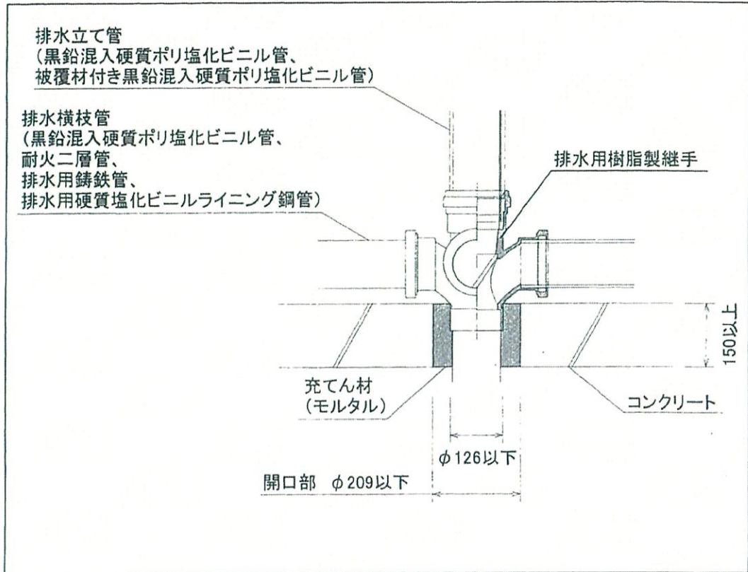
図6 施工図例
