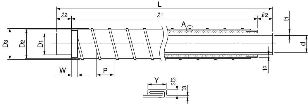
A 部詳細
